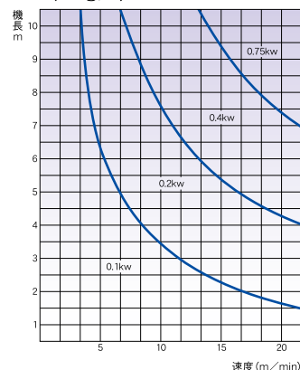
■ 機長・速度・出力の組合せ目安表 (50kg/m)
